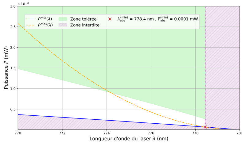
FIGURE 7.6 – Puissance requise en fonction de la longueur d'onde pour w_0 = 1 \mu m
